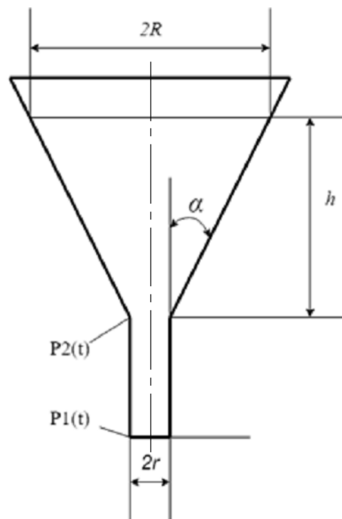
Рис.4. Бункер конічної форми
