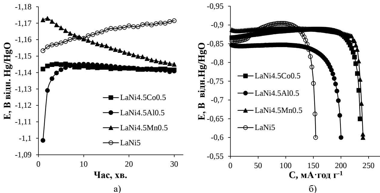
Рис. 2. Хронопотенціометричні криві контактного заряду електродів складу \text{LaNi}_{5-x}\text{M}_x (а) та гальваностатичне визначення ефективності такого заряду (б)
