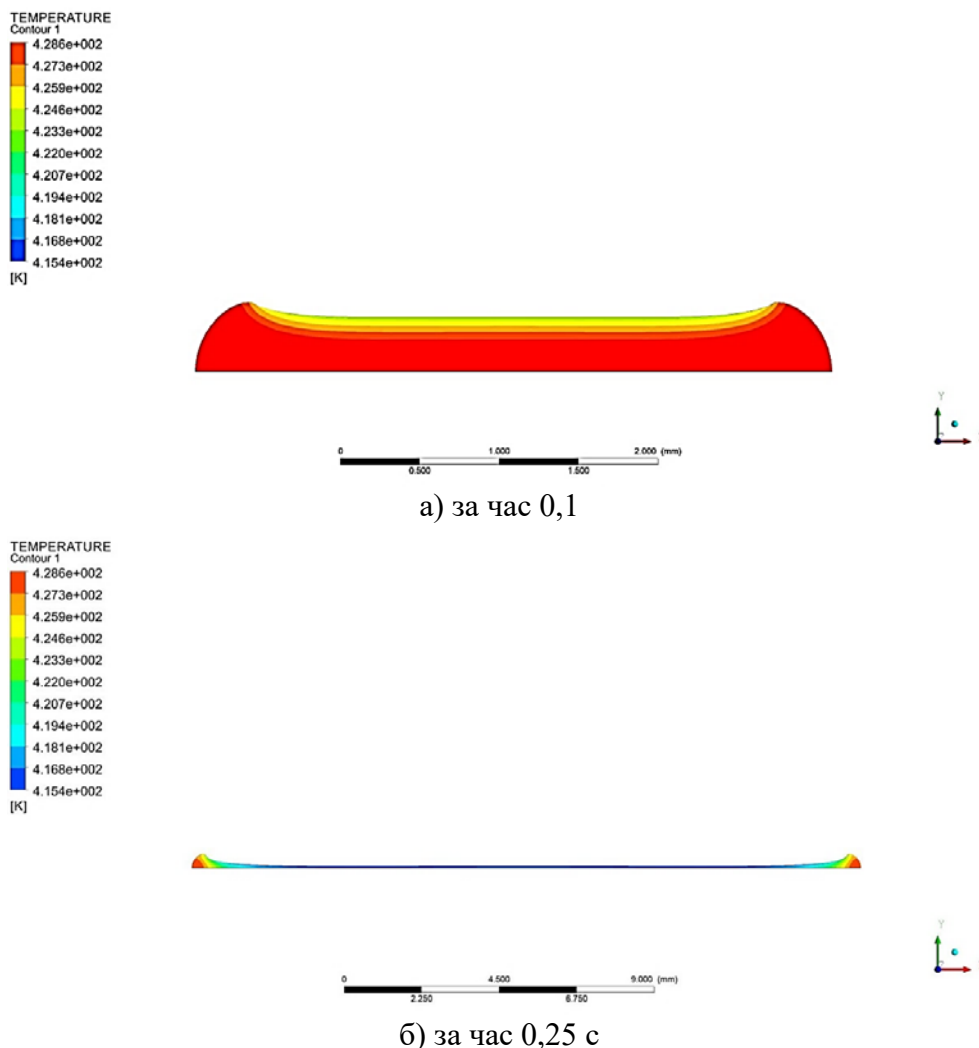
Рис. 5. Розподіл температур та форма шару термоклею при притискному зусиллі валків 21,66 Н
