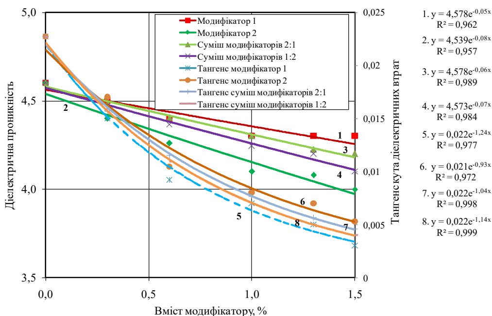
Рис.8. Залежність діелектричної проникності та тангенсу кута від вмісту модифікаторів, для полімерних композицій на основі КЕВ-2 та антипірену 2:крива 1,5 – модифікатор 1, крива 2,6 – модифікатор 2,крива 3,7 – суміш модифікаторів де, k_1 = 0,67 ; k_2 = 0,33 ; крива 4,8 – суміш модифікаторів де, k_1 = 0,33 ; k_2 = 0,67 ;
