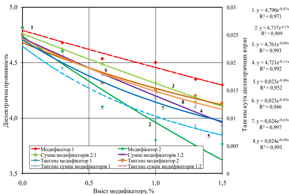
Рис.7. Залежність діелектричної проникності та тангенсу кута від вмісту модифікаторів, для полімерних композицій на основі КЕВ-2 та антипірену 1:крива 1,5 – модифікатор 1, крива 2,6 – модифікатор 2,крива 3,7 – суміш модифікаторів де, k_1 = 0,67 ; k_2 = 0,33 ; крива 4,8 – суміш модифікаторів де, k_1 = 0,33 ; k_2 = 0,67
