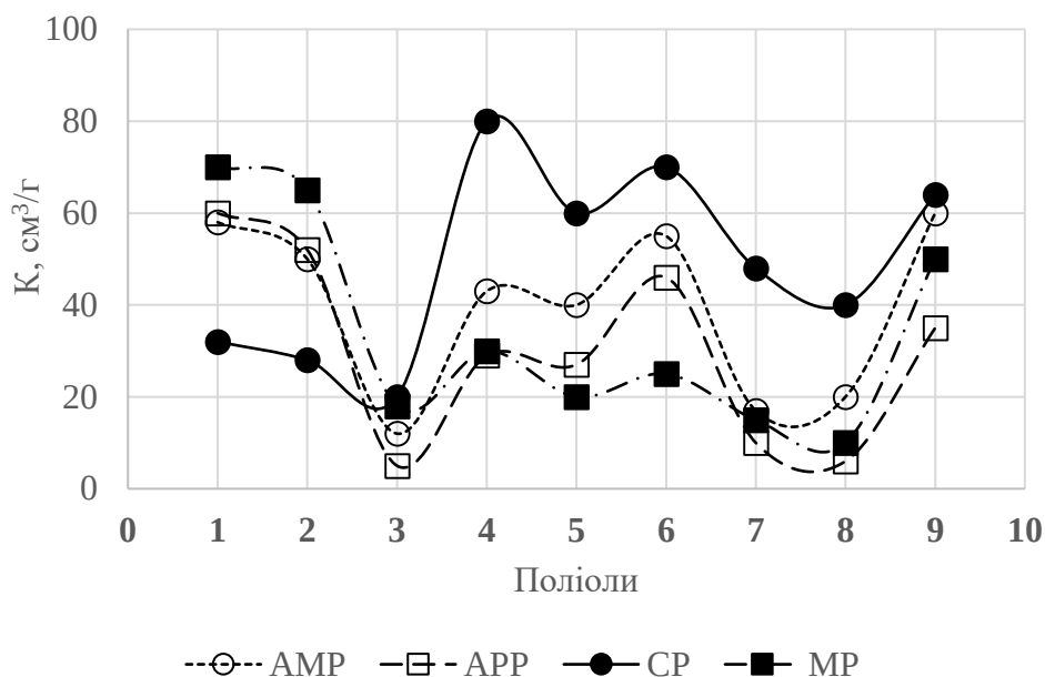
Рис. 1. Значення коефіцієнта спучення ( K , \text{см}^3/\text{г} ) для різних поліолів: система донор кислоти/поліол при співвідношенні 3:1 (за мас.); поліол: пентаеритрит (1), дипентаеритрит (2), триметилпропан (3), крохмаль (4), декстрин (5), ксиліт (6), глюкоза (7), цукроза (8), сорбіт (9); донор кислоти: моноамоній фосфат (AMP), поліамоній фосфат (APP), меламін фосфат (MP)
