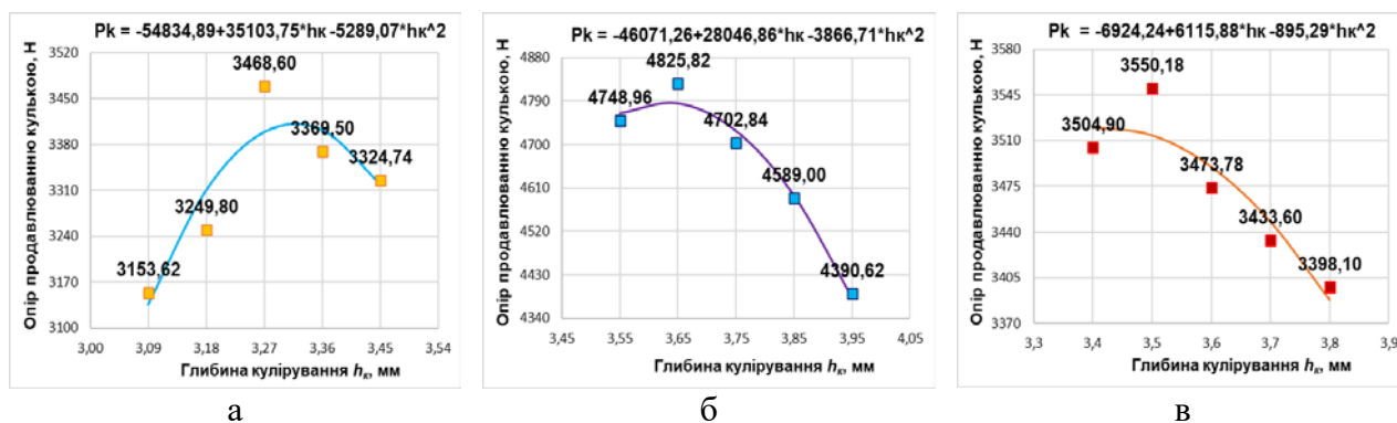
Рис. 5. Графіки залежності величини зусилля продавлювання кулькою від зміни щільності в'язання: з UHMWPE нитки: а) з платинами РА; з pA нитки: б) без платин ПВРК; в) з платинами РА
