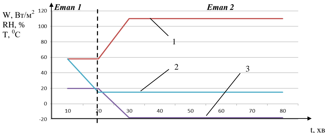
Рис. 1. Умови проведення порівняльних тестувань: 1 – енерговитрати суб'єкту W, Вт/м 2 ; 2 – відносна вологість навколишнього середовища RH, %; 2 – температура навколишнього середовища T, °C
