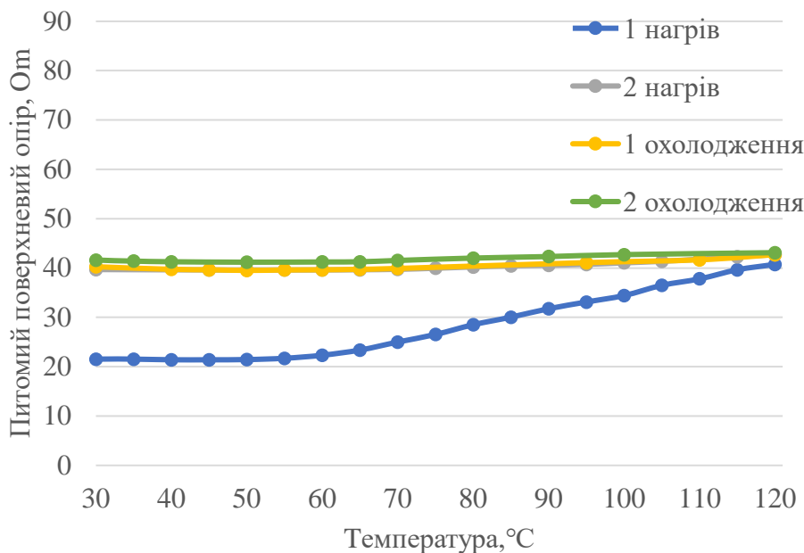
Рис. 2. Залежність питомого поверхневого електричного опору від температури для композиції №1
