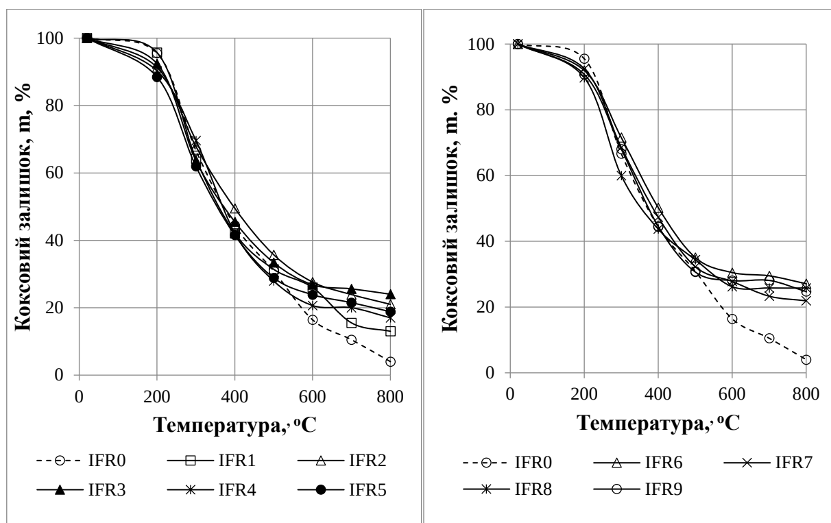
Рис. 1. Залежність маси коксового залишку m (%) інтумесцентних композицій від температури T (°C)
