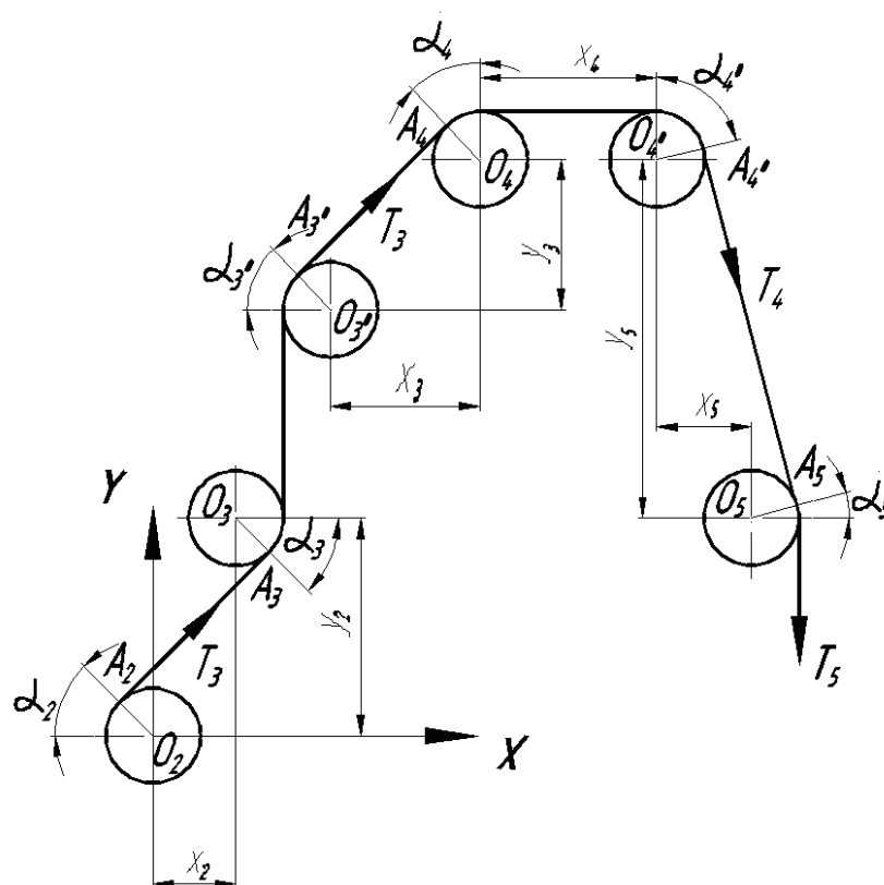
Рис. 2. Розрахункова схема системи пасивної подачі ниток: 2, 3, 3', 4, 4', 5 – вічка нитконапрямлячі; \alpha_2, \alpha_3, \alpha_4, \alpha_{4'}, \alpha_5 – кути обхвату; T_i – натяги нитки на ділянках заправної лінії; x_i та y_i – горизонтальні та вертикальні відстані між осями вічок; O_2, O_3, O_{3'}, O_4, O_{4'} та O_5 – центри циліндричних поверхонь вічок
