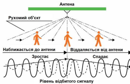
Рис. 6. Мікрохвильові датчики
