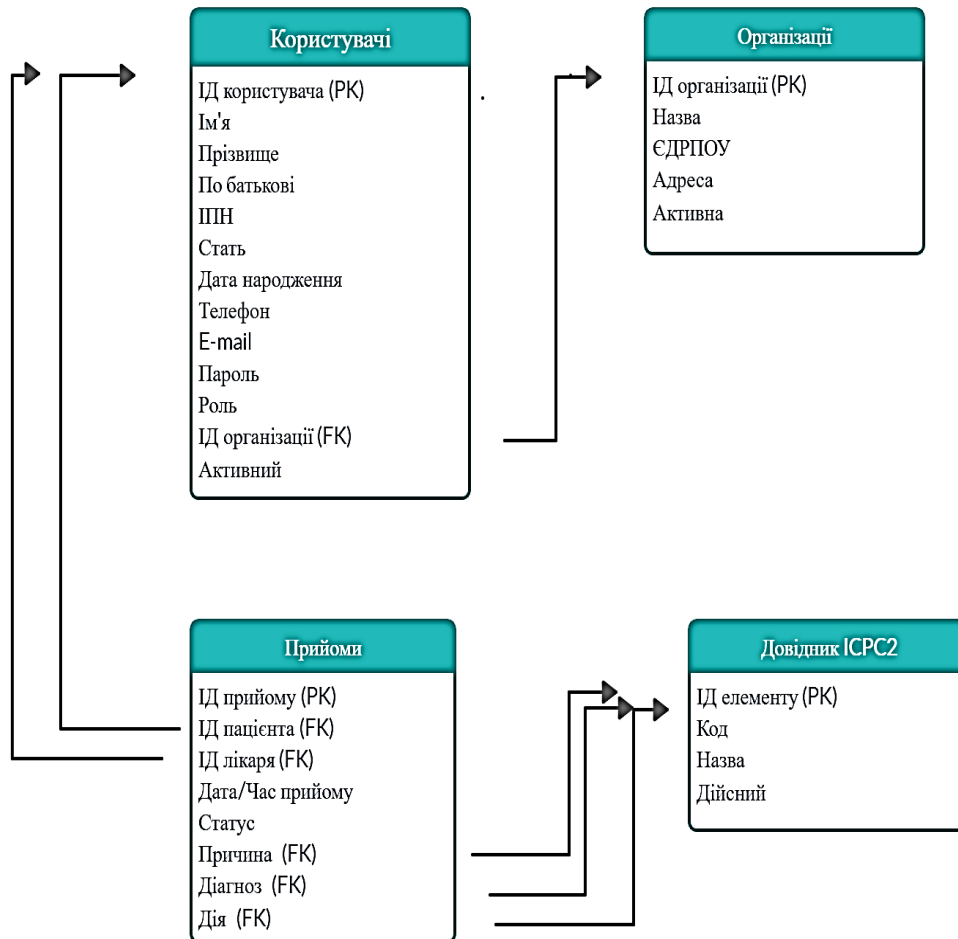
Рис. 2. Схема бази даних
