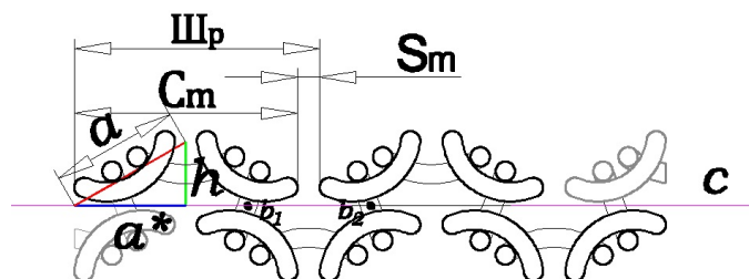
Рис. 1. Переплетення ластик 2х2 в умовно-рівноважному стані
