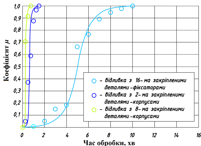
Рис. 2. Залежність коефіцієнту \mu від часу обробки при обробці відливок різного типу
