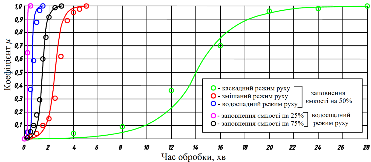
Рис. 2. Залежність коефіцієнта \mu від часу обробки при реалізації різних режимів руху робочого масиву та різних ступенях заповнення ємкості
