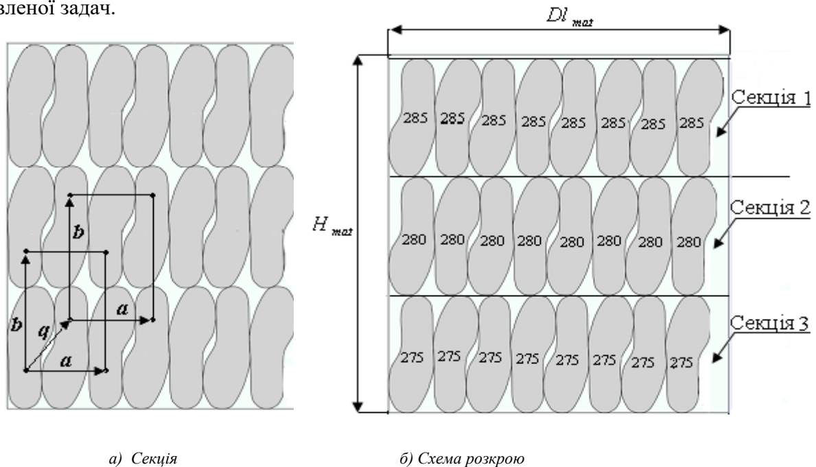
Рис. 1. Секція та схема розкрою
