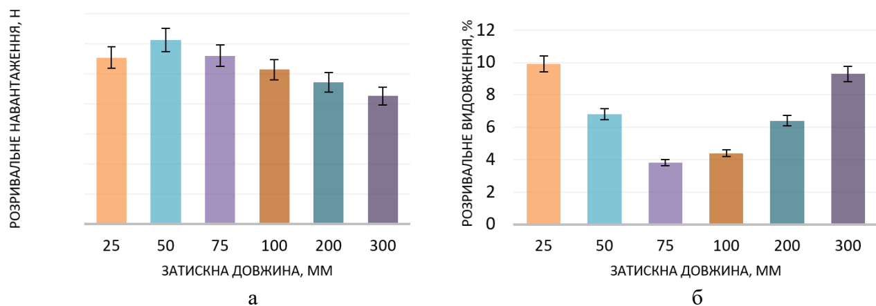
Рис. 2. Діаграми розривального зусилля (а) та видовження (б) при заправці у затискачі 6 рА ниток лінійної густини 44 текс
