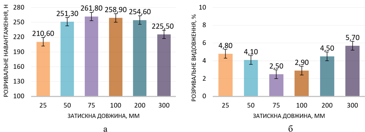
Рис. 3. Діаграми розривального зусилля (а) та видовження (б) при заправці петлею рА нитки лінійної густини 44 текс×3
