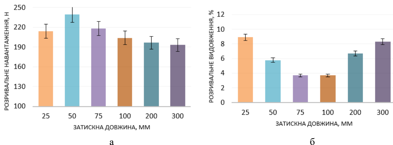
Рис. 1. Діаграми розривального зусилля (а) та видовження (б) при заправці у затискачі 3 рА ниток лінійної густини 44 текс
