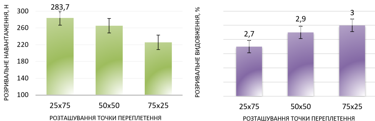
Рис. 5. Діаграми розривального зусилля (а) та видовження (б) при заправці у затискачі pA нитки лінійної густини 44 текс×3 петлею
