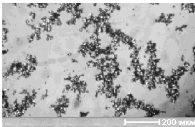
Рис. 1. Мікрофотографія зольного залишку після термічної обробки сажі «VULCAN Р»
