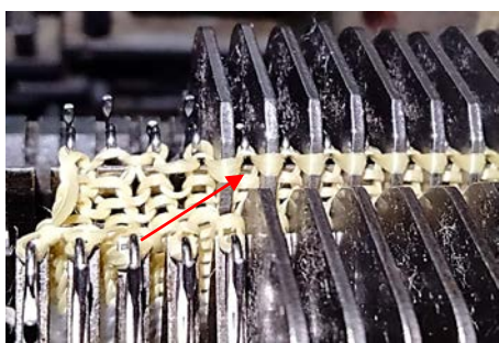
Рис. 2. Процес формування петель на плосков'язальному рукавичковому автоматі ПА-8-33: відбійною площиною слугують підборіддя платин
