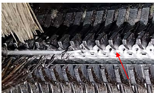
Рис. 1. Процес формування петель на плосков'язальній машині типу ПВРК 8 класу: відбійною площиною слугують відбійні зубці голечниці
