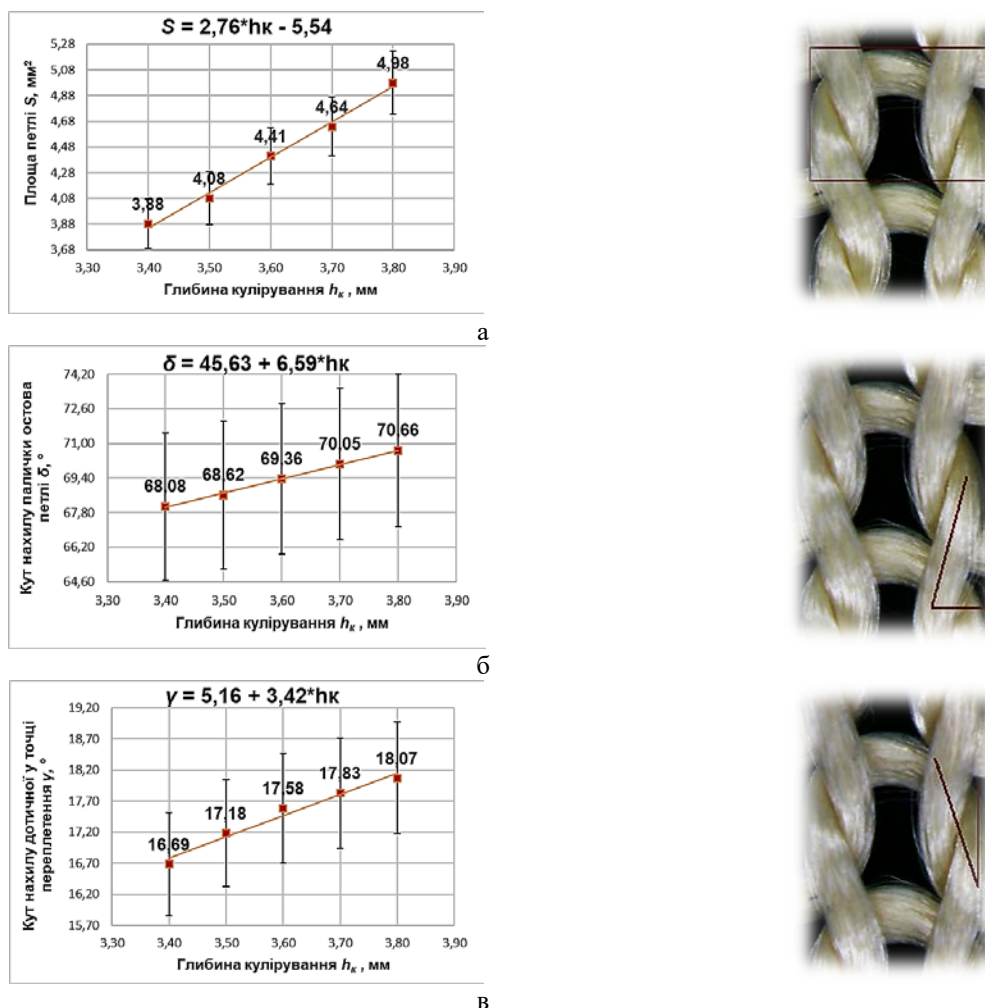
Рис. 6. Макрофотографії та графіки залежності характеристик формоутворення петель в структурі трикотажу, виробленого з пара-арамідних ниток, від зміни глибини кулірування: а – площа петлі трикотажу; б – кут нахилу паличок остова петлі трикотажу; в – кут нахилу дотичної у точці переплетення ниток в петлі трикотажу
