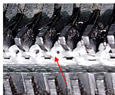
Рис. 1. Процес формування петель на плосков'язальній машині типу ПВРК 8 класу: відбійною площиною слугують відбійні зубці голечниці
