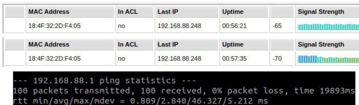
Рис. 6. Результат перевірки якості каналу при рівні сигналу у -65...-70 дБм
