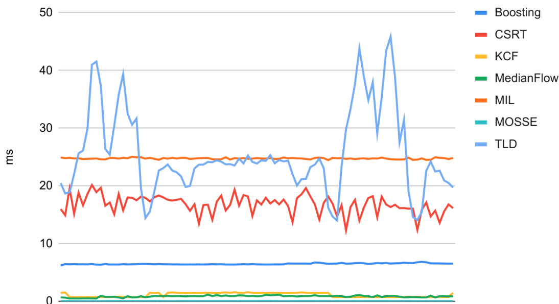
Рис. 22. Збільшення витрат часу TLD під час спотворення зображення
