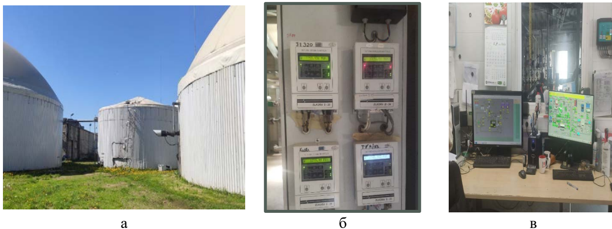
Рис. 1. Біогазові установки, в яких відбуваються послідовні процеси ферментації: а – біогазові установки, б – датчики контролю за процесом ферментації, в – пункт оператора (автоматичний контроль процесу ферментації відходів)
